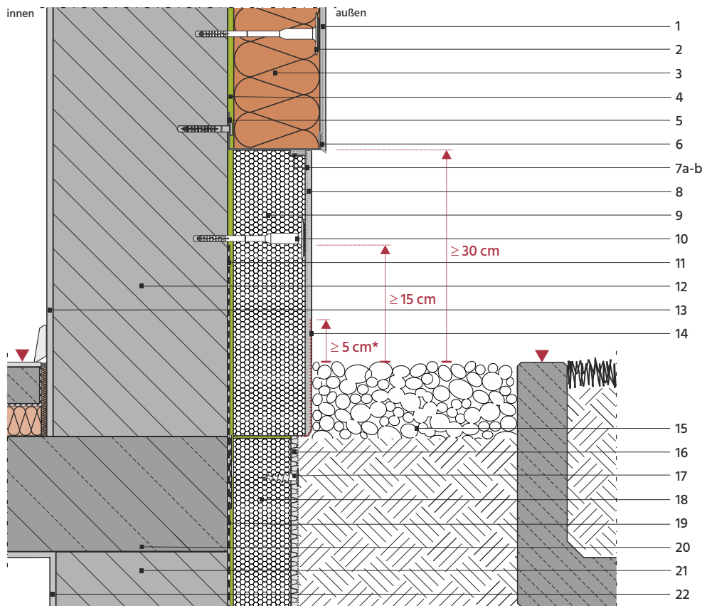
Vertikalschnitt M 1:7,5
